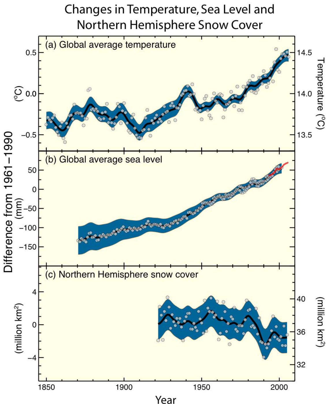
Obrázek SPM-3. Pozorované změny (a) globální průměrné teploty vzduchu při zemském povrchu; (b) globálního průměrného zvýšení mořské hladiny na základě přímých přístrojových měření výšky hladiny (modrá) a družicových měření (červená) a (c) rozsahu sněhové pokrývky na severní polokouli v období březen–duben. Všechny změny jsou udávány jako odchylky od průměrů za období 1961–1990. Shlazené křivky představují desetileté průměrné hodnoty zatímco kroužky znázorňují roční hodnoty. Vyplněné oblasti představují intervaly neurčitosti odhadnuté pomocí rozsáhlé analýzy známých neurčitostí (a a b) a z časových řad (c). {FAQ 3.1, Obrázek 1, Obrázek 4.2, Obrázek 5.13}
