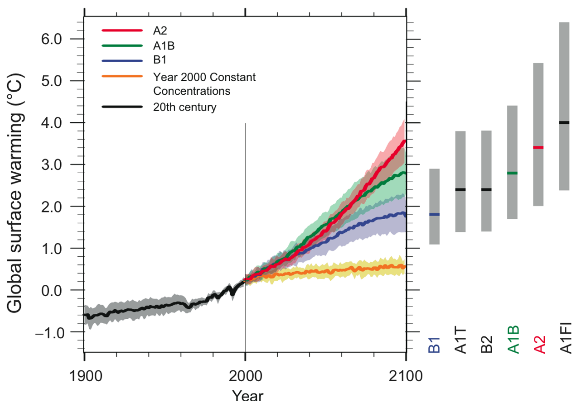
Obrázek SPM-5. Nepřerušované čáry představují průměry globálního oteplování zemského povrchu (ve srovnání s obdobím 1980-99) vypočítané z mnoha klimatických modelů pro scénáře A2, A1B a B1 a znázorněné jako prodloužení simulací pro 20. století. Vybarvená oblast odpovídá rozsahu plus minus jedné směrodatné odchylky vypočítané z ročních průměrů pro jednotlivé modely. Oranžová čára představuje experiment, při kterém byly koncentrace udržovány konstantní na úrovni roku 2000. Šedé sloupce v pravé části obrázku ukazují nejlepší odhad (vodorovná čárka uvnitř každého sloupce) a pravděpodobný rozsah hodnot získaný pro každý ze šesti scénářů SRES. Při stanovení nejlepších odhadů a pravděpodobných intervalů (šedé sloupce) byly v levé části obrázku použity modely typu AOGCM a též výsledky získané z hierarchie nezávislých modelů a pozorování. {Obrázky 10.4 a 10.29}
