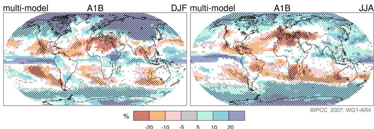
Obrázek SPM-7. Relativní změna srážek (%) pro období 2090-2099 ve srovnání s obdobím 1980-1999. Hodnoty představují vícemodelový průměr založený na scénáři SRES A1B pro prosinec až únor (vlevo) a červen až srpen (vpravo). Bíle jsou znázorněny oblasti, kde se méně než 66 % modelů shoduje na znaménku změny; tečkované oblasti, kde se na znaménku změny shoduje více než 90 % modelů. {Obrázek 10.9}
