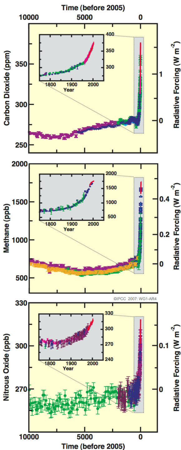
Obrázek SPM-1. Atmosférické koncentrace oxidu uhličitého, metanu a oxidu dusného za posledních 10 000 let (velké panely) a od roku 1750 (vnořené panely). Jsou znázorněna měření z ledovcových vrtů (symboly různých barev značí různé studie) a atmosférická měření (červená čára). Odpovídající hodnoty radiačního působení jsou vyneseny na pravé straně velkých panelů.
